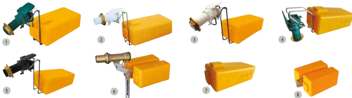
Certains robinets flotteurs sont équipés d'une vis de réglage hauteur d'eau/débit.
